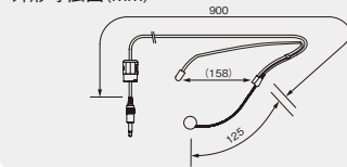
外形寸法図(mm)
