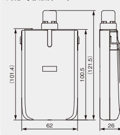
外形寸法図(mm)
