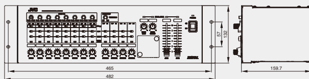
外形寸法図(mm)
