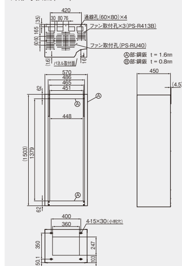
外形寸法図(mm)
