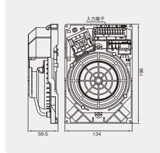
外形寸法図 (mm)
