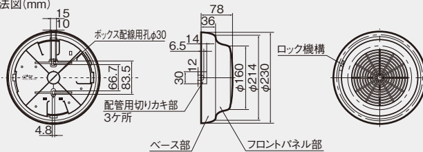
外形寸法図(mm)
