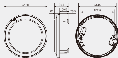
外形寸法図(mm)
