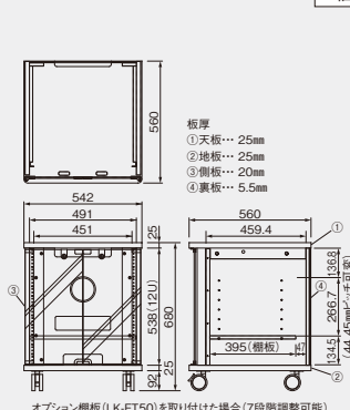
外形寸法図(mm)
