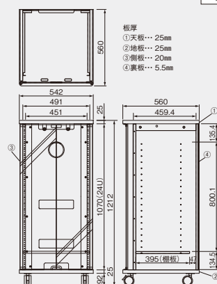
外形寸法図(mm)
