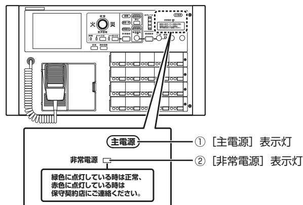
非常業務遠隔操作器（EM-C156）
