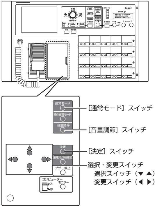
非常業務遠隔操作器 (EM-C156)
