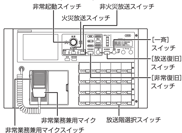
非常業務遠隔操作器 (EM-C156)
