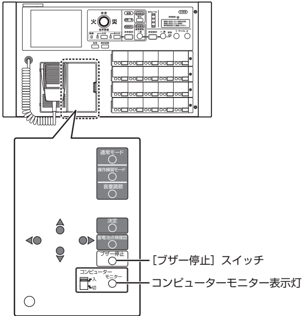
非常業務遠隔操作器（EM-C156）
