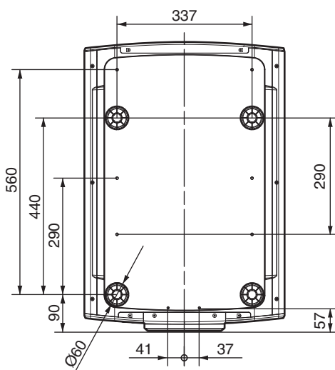
底面
