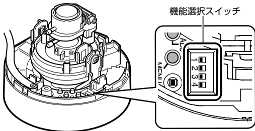
機能選択スイッチの設定表
