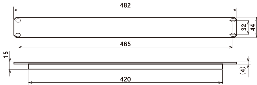
パネル取付穴寸法
