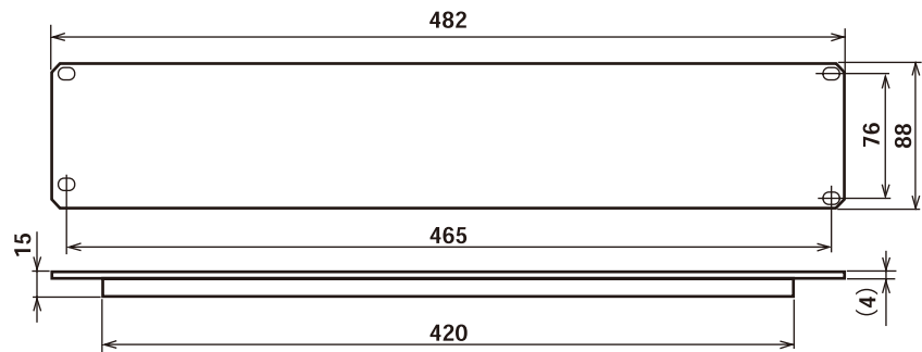
パネル取付穴寸法
