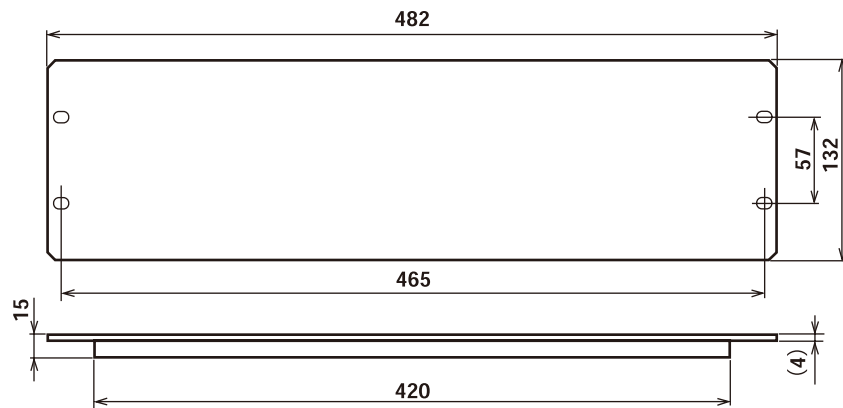
パネル取付穴寸法
