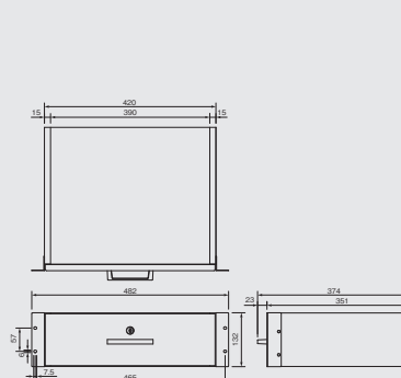
外形寸法図(mm)
