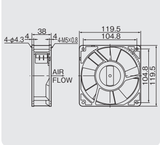
外形寸法図(mm)
