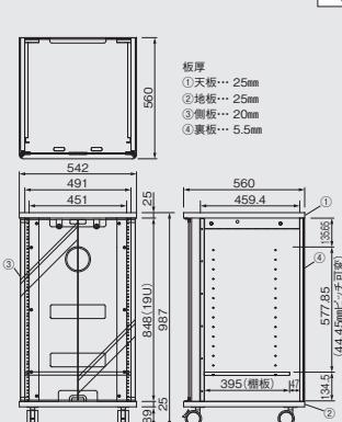
外形寸法図(mm)
