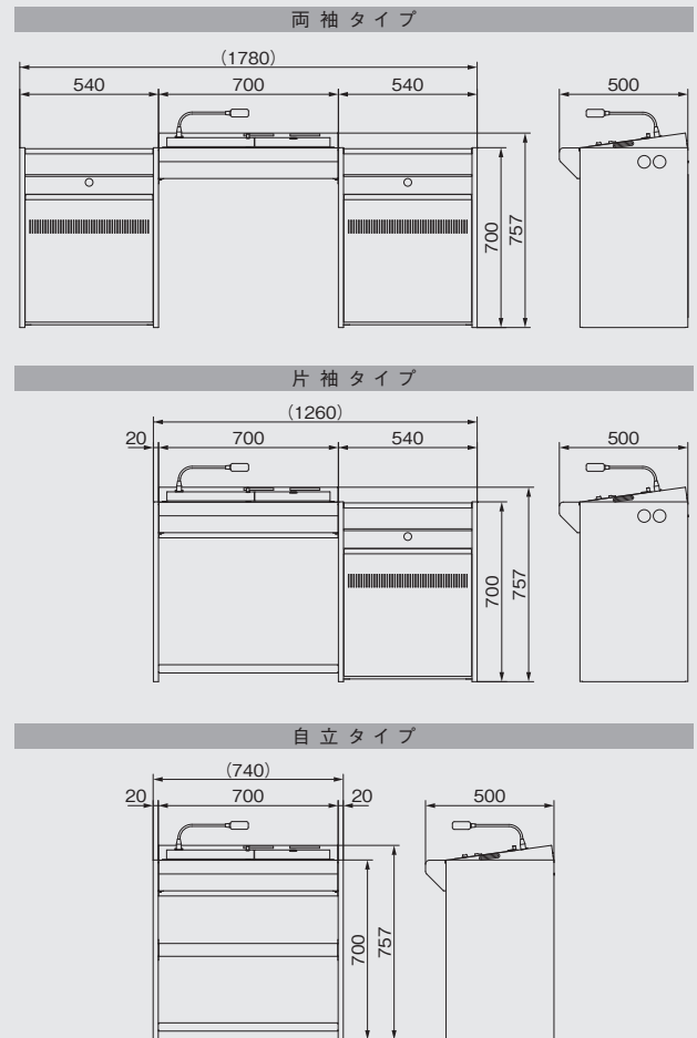
外形寸法図(mm)
