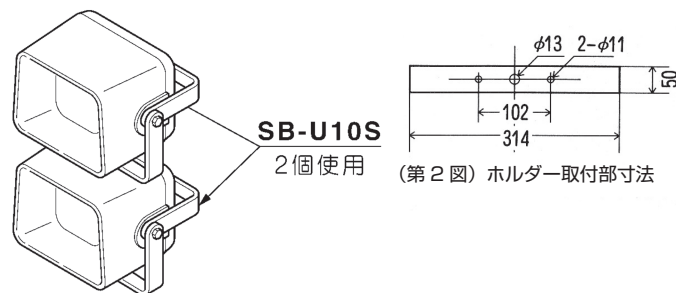
(第1図) 2台スタックの場合の使用数 SB-U10S…2ヶ
