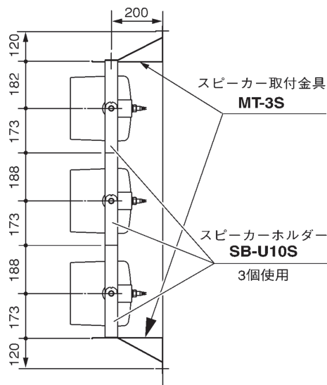
(第3図) 3台スタッキング時の寸法
